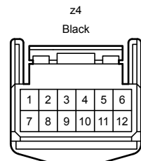
90980-12559
