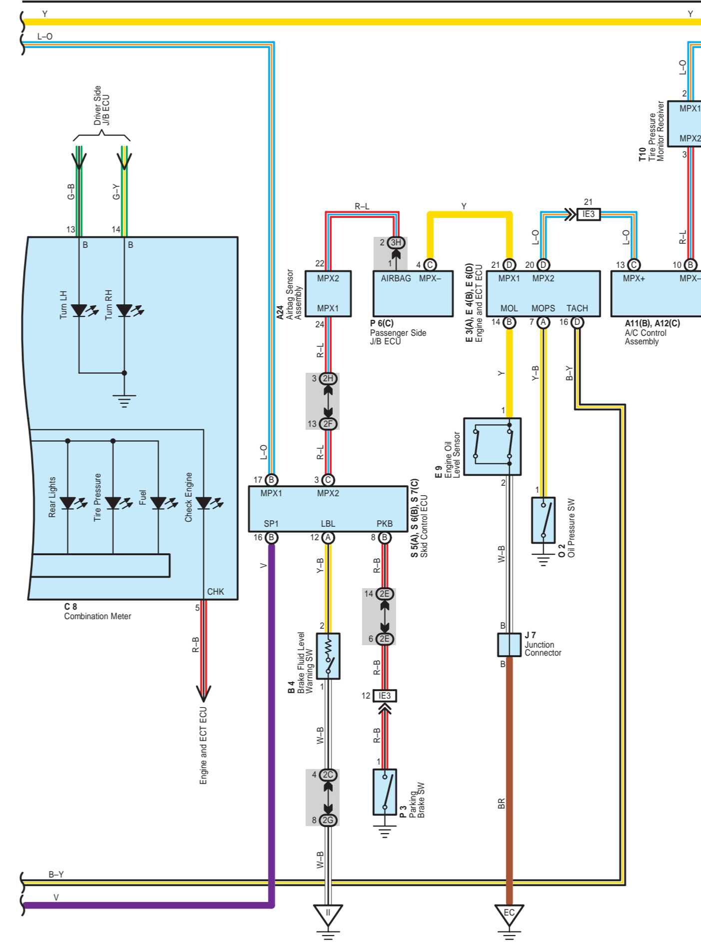
LEXUS SC 430 (EWD447E)
