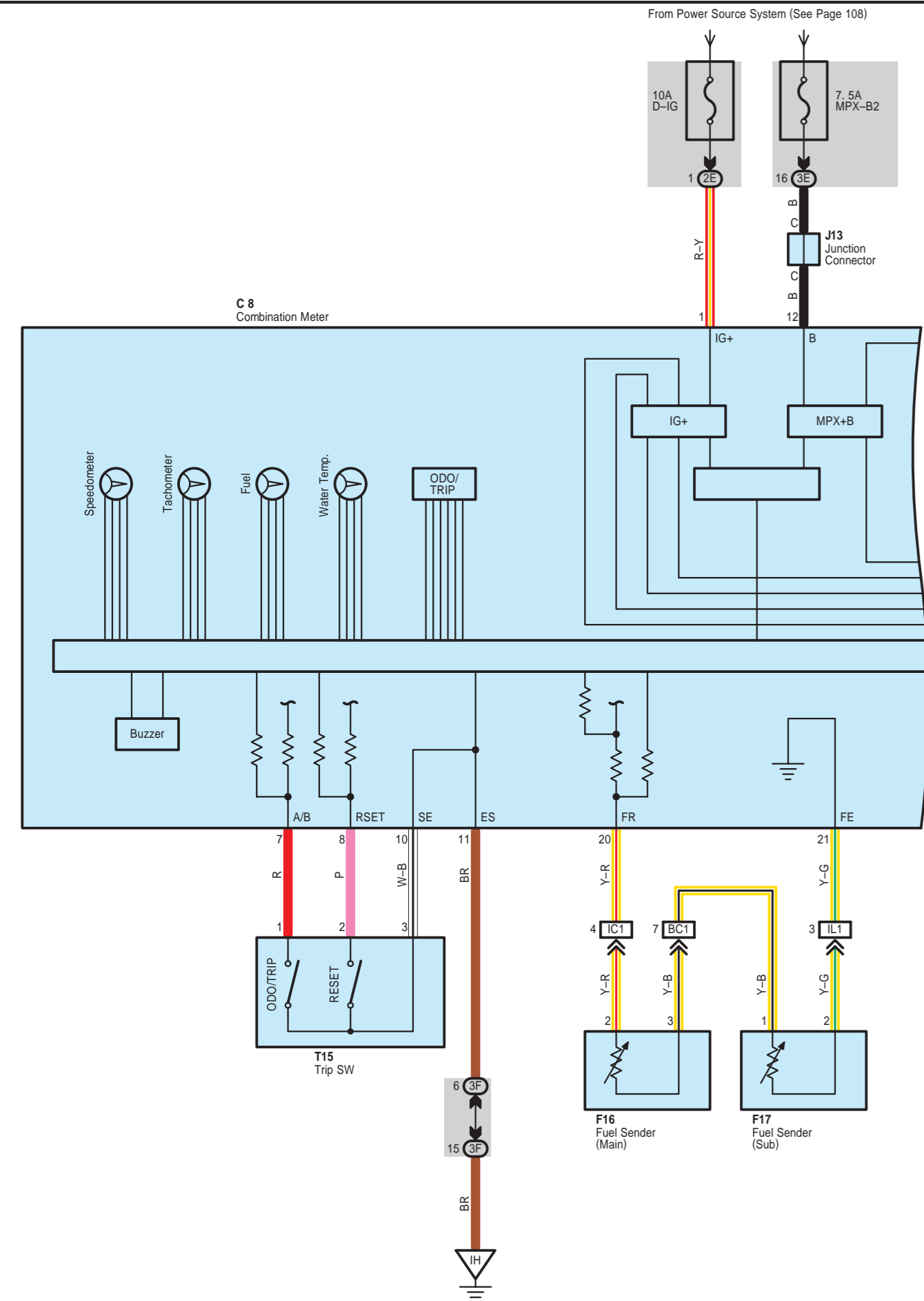
LEXUS SC 430 (EWD447E)
